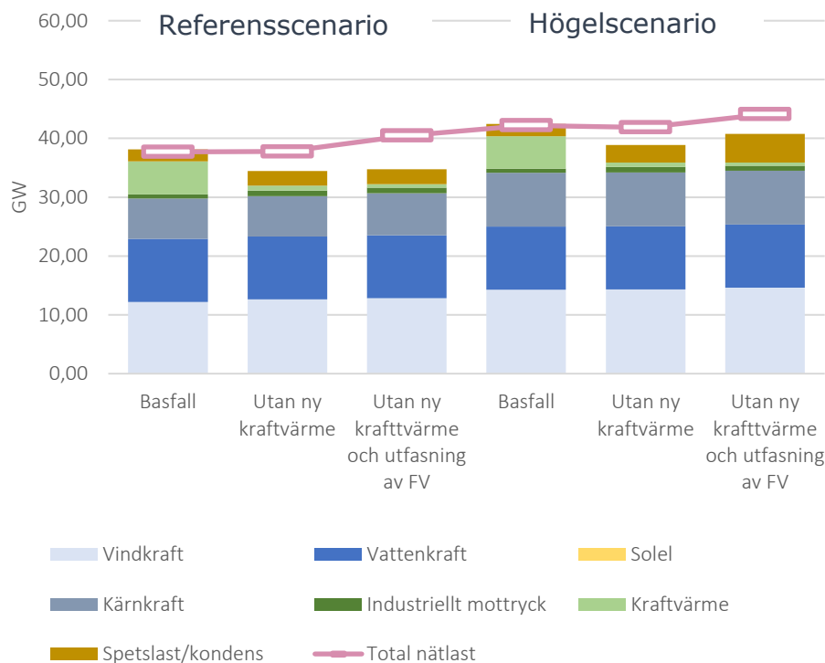
Figur 10 Eleffektbalansen under vinterdagseftermiddagen olika beräkningsfall (modellår 2040).
